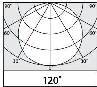
配光データ
